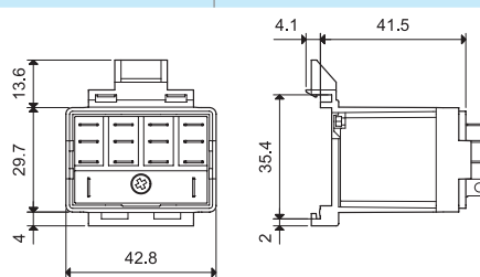
056.47 con relé
