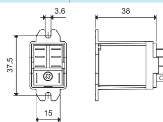
056.25 con relé
