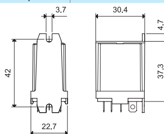
056.26 con relé
