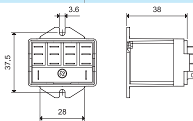
056.45 con relé
